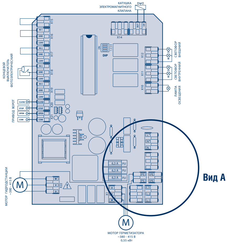
Рис. 5.2.1. Вид А. Подключение источника питания
